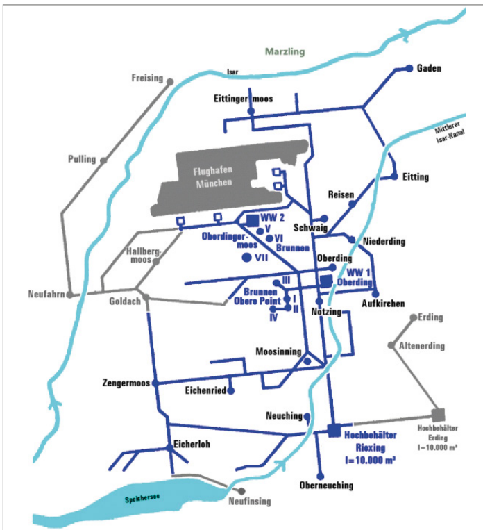
Hauptleitungsstruktur
